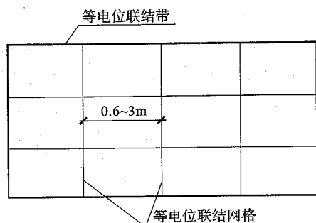
图1 等电位联结带与等电位联结网格
